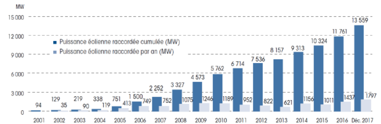
Evolution de la puissance éolienne raccordée entre 2001 et 2017 1 .
